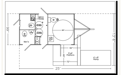
Floorplan · 2 Stalls + ADA
