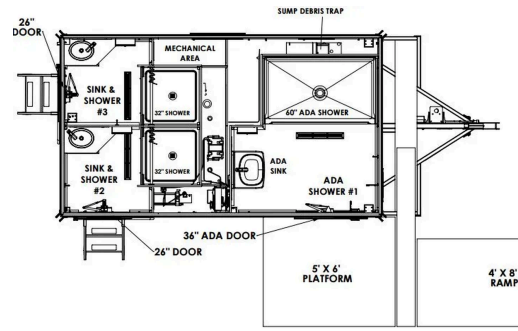
Floorplan · 2 Showers + ADA
