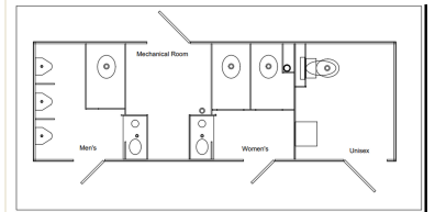
Floorplan · 6 Stalls + ADA
