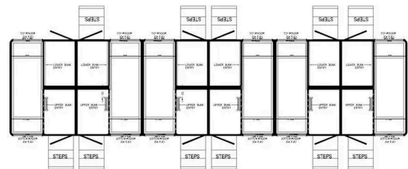
Floorplan · 12 Bunks
